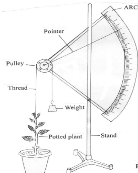
Fig. 19.3 Auxanometer
